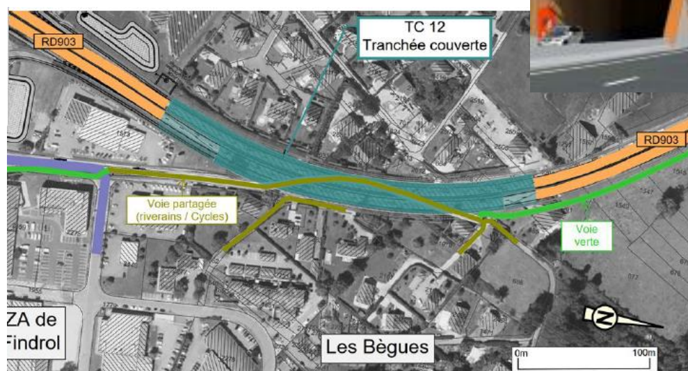
Fig.4 : Tranchée couverte
